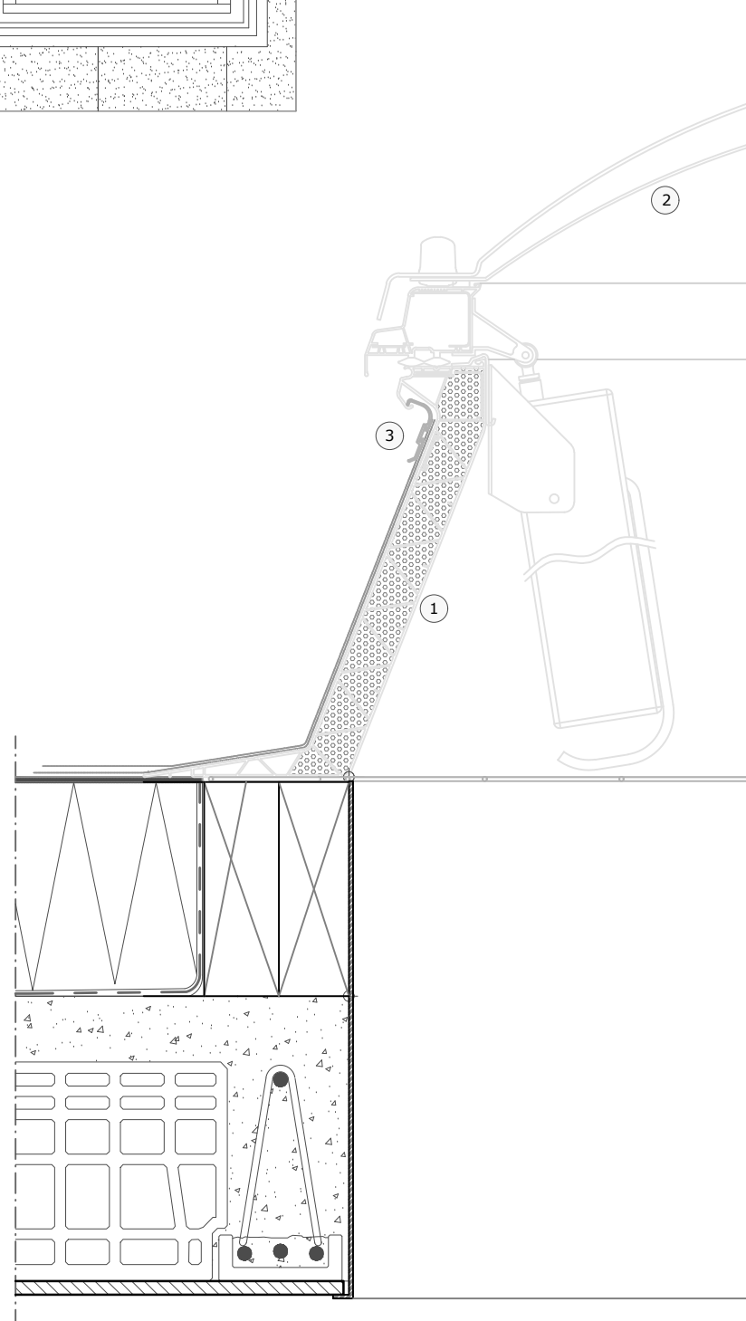
Presek A-A 1:5
